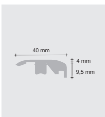
Cantonera de escalón, plana Para un acabado enrasado en los peldaños de las escaleras.
